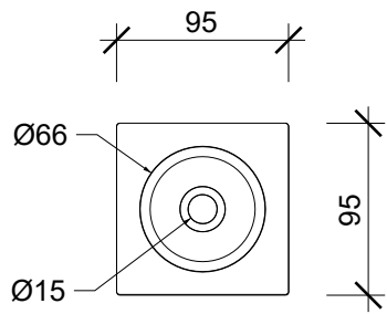
Obenansicht top view
