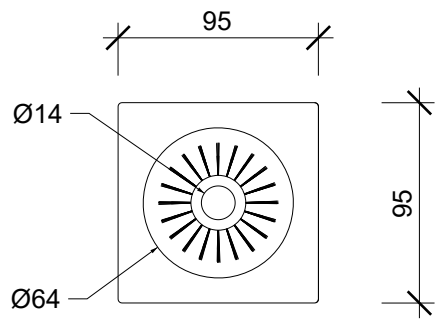
Obenansicht top view
