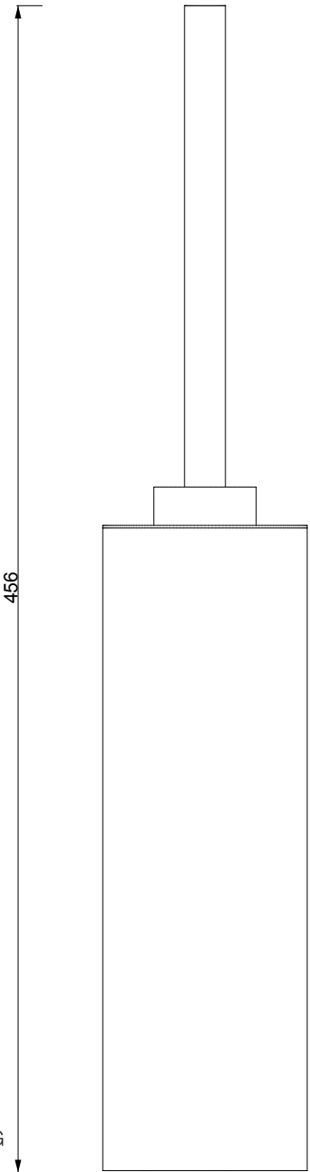
Seitenansicht - CENTURY SBG Side view - CENTURY SBG
